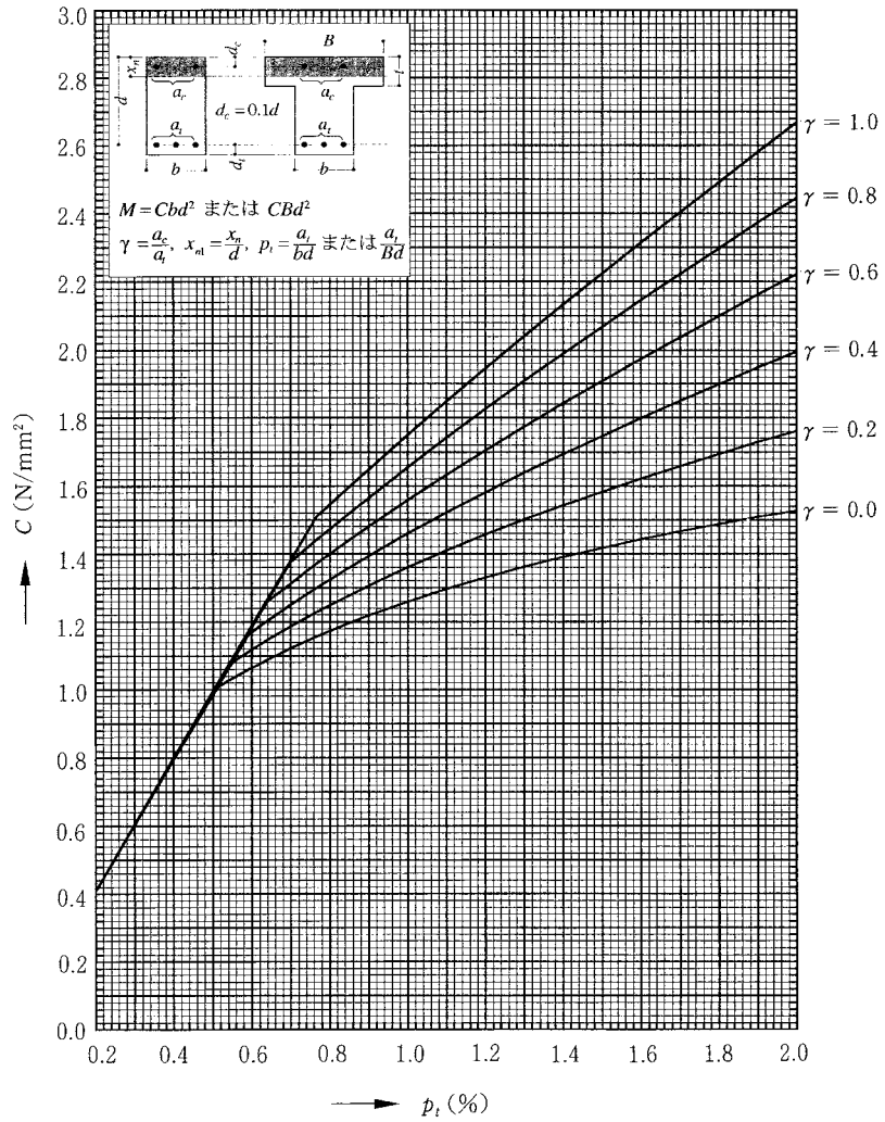
長方形梁およびT形梁 (中立軸スラブ内) (2)
