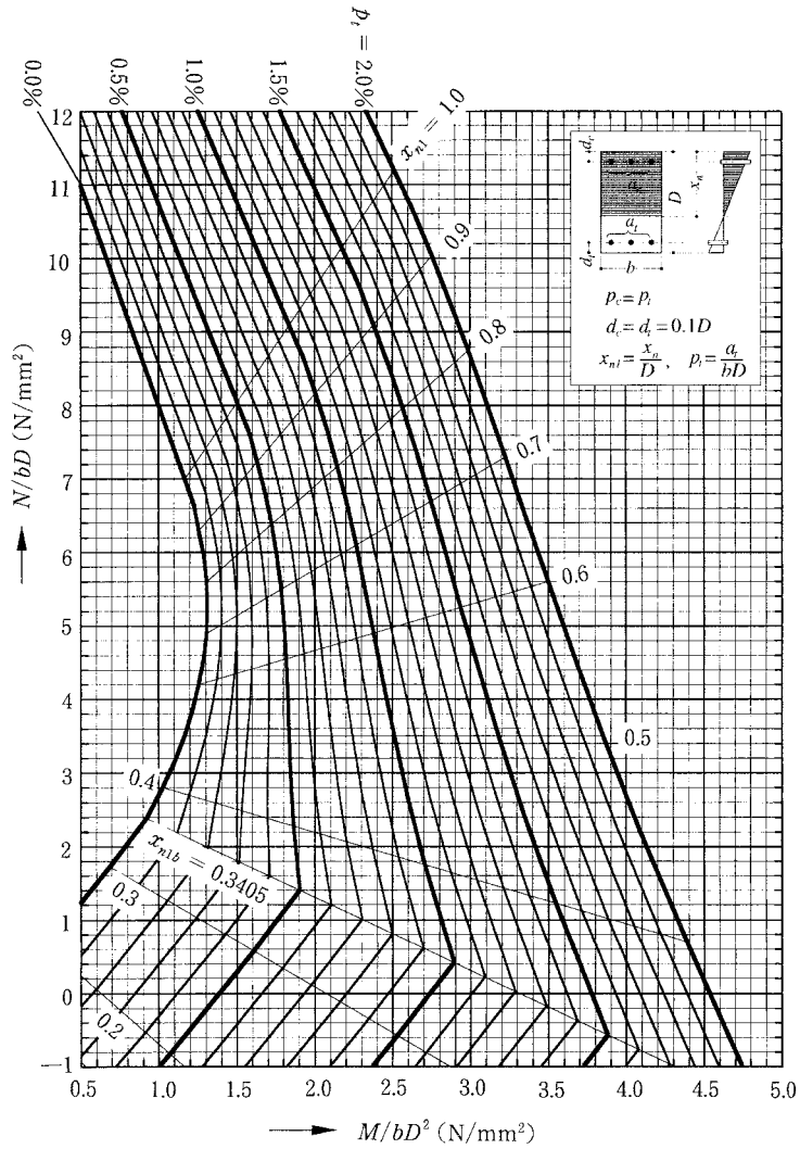
長方形断面柱
